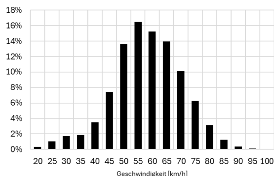
Geschwindigkeitsverteilung der erfassten Fahrzeuge bei der Volksschule Nappersdorf
